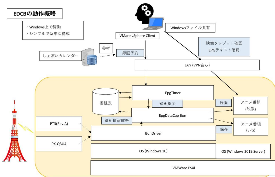
図 3-3 全録サーバ (杉並) のシステム構成図
