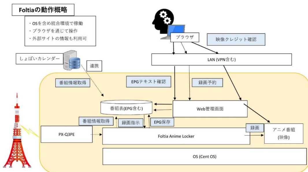
図 3-6 全録サーバ (千代田) のシステム構成図
