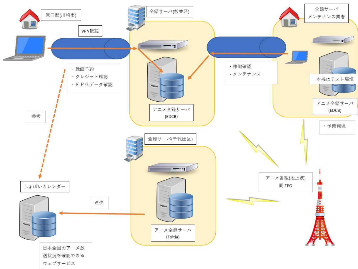
図 3-2 全録サーバ (2 種) のシステム概要
